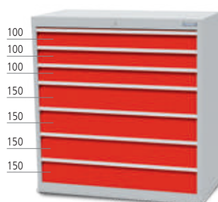
■ 7 x Schublade
